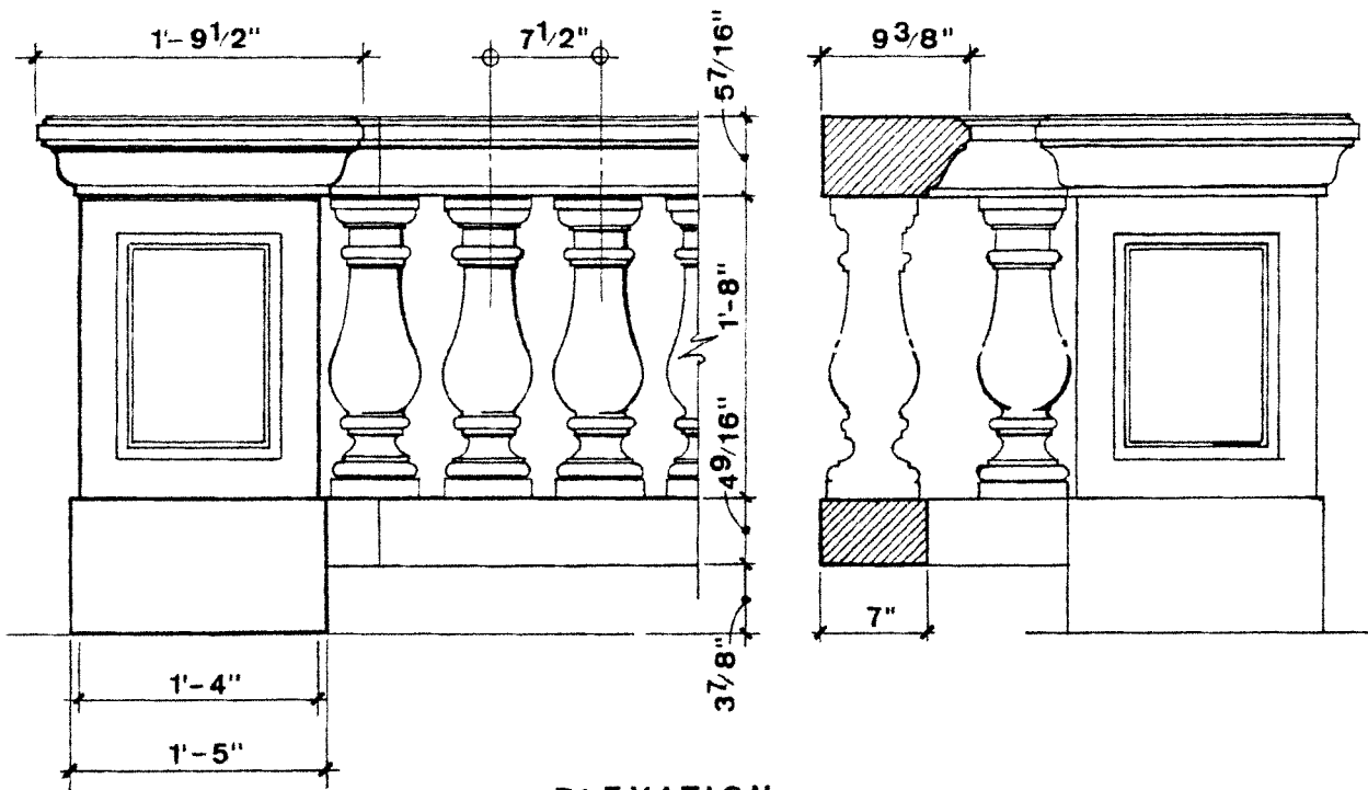
ELEVATION
