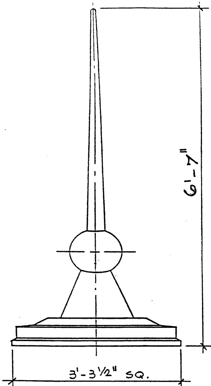
ELEVATION
